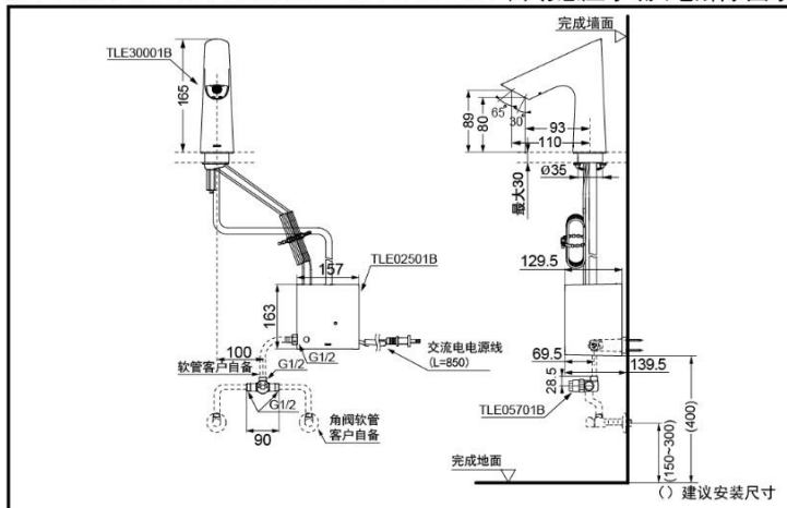
TLE30001B+TLE02501B+TLE05701B 自动感应水嘴(电解除菌水型)+控制器部(恒温)
