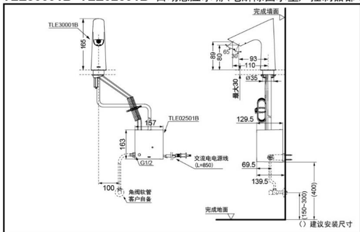
TLE30001B+TLE02501B 自动感应水嘴(电解除菌水型)+控制器部(单冷)
